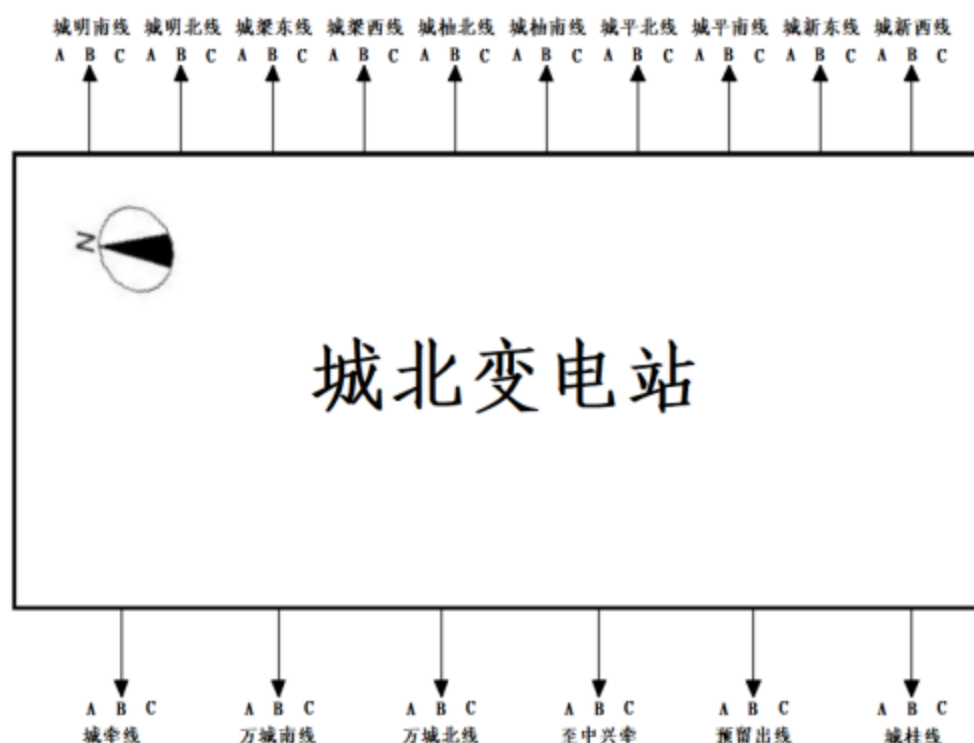
图 2-1 220kV 城北变电站间隔情况
